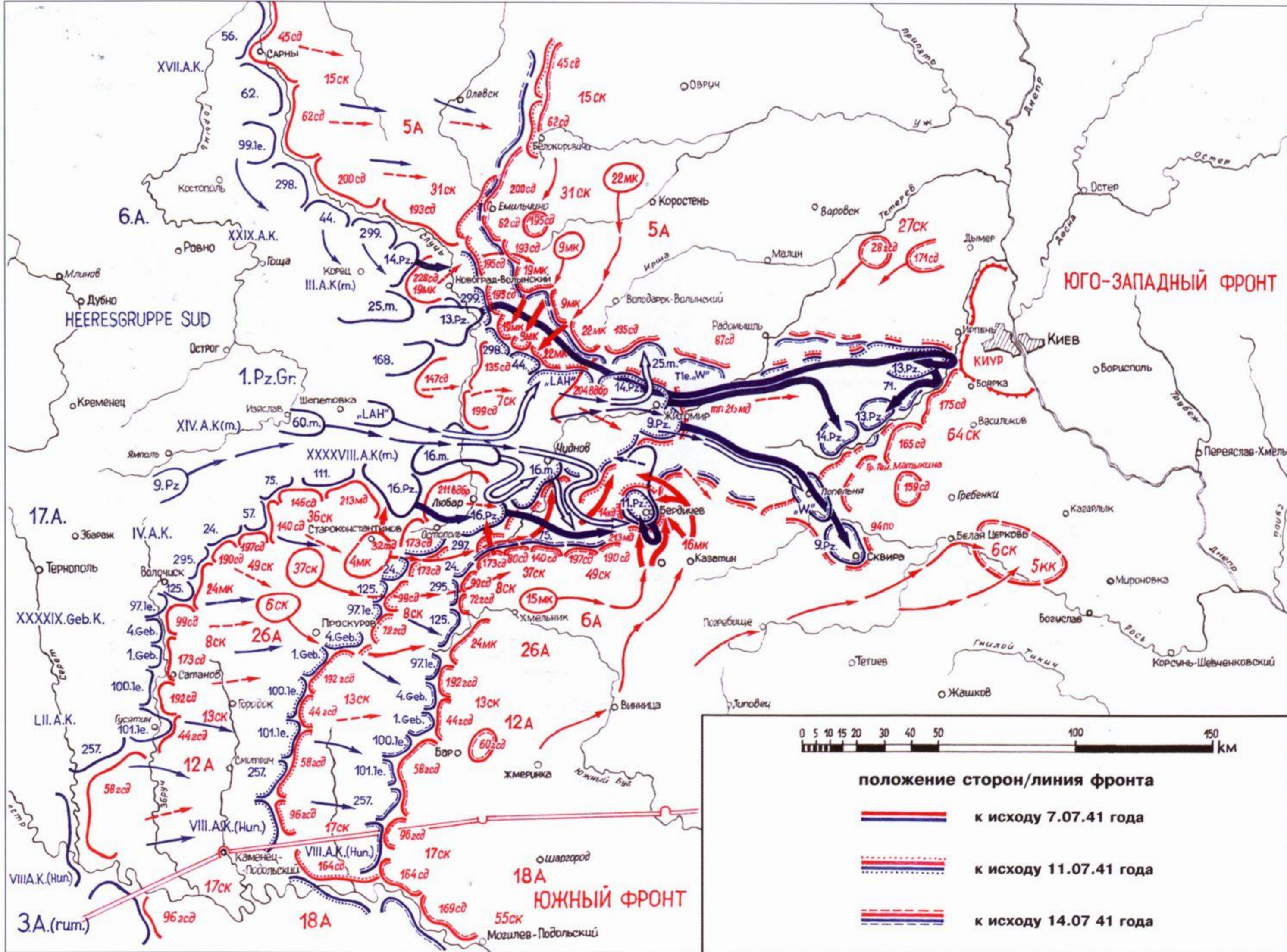
Действия войск Юго-Западного фронта в первой половине июля 1941 года. Operations of troops of the South-Western Front in July 1941.
